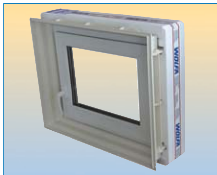
Ościeżnica typu ZOW z wysokiej jakości wkładem okiennym o profilu 3- lub 5-komorowym z szybą ciepłoszczelną Ug 1, 1 zgodną z aktualnymi standardami EnEV i wytycznymi RAL.
