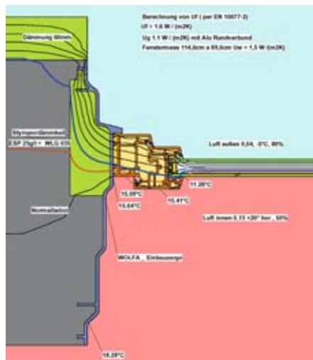
Okno uchylno-otwieralne typu MDK z profilem 3-komorowym jako wkład do ościeżnicy
